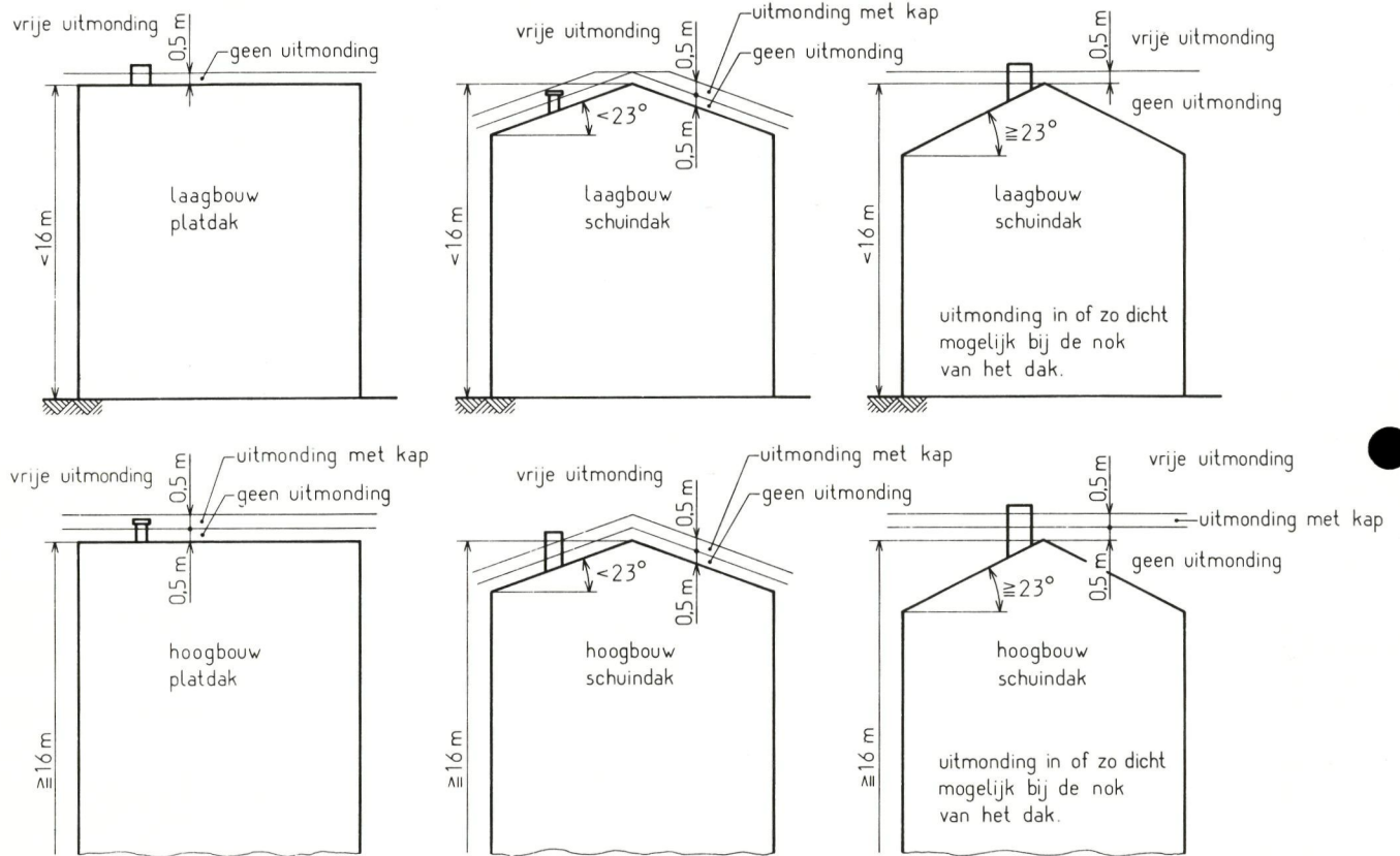
Uitmondning van een afvoerkanaal of afvoerleiding ten opzichte van het eigen dakvlak.
