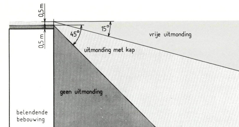
Uitmondning van een afvoerkanaal of afvoerleiding, in verband met goede werking en met hinder.
